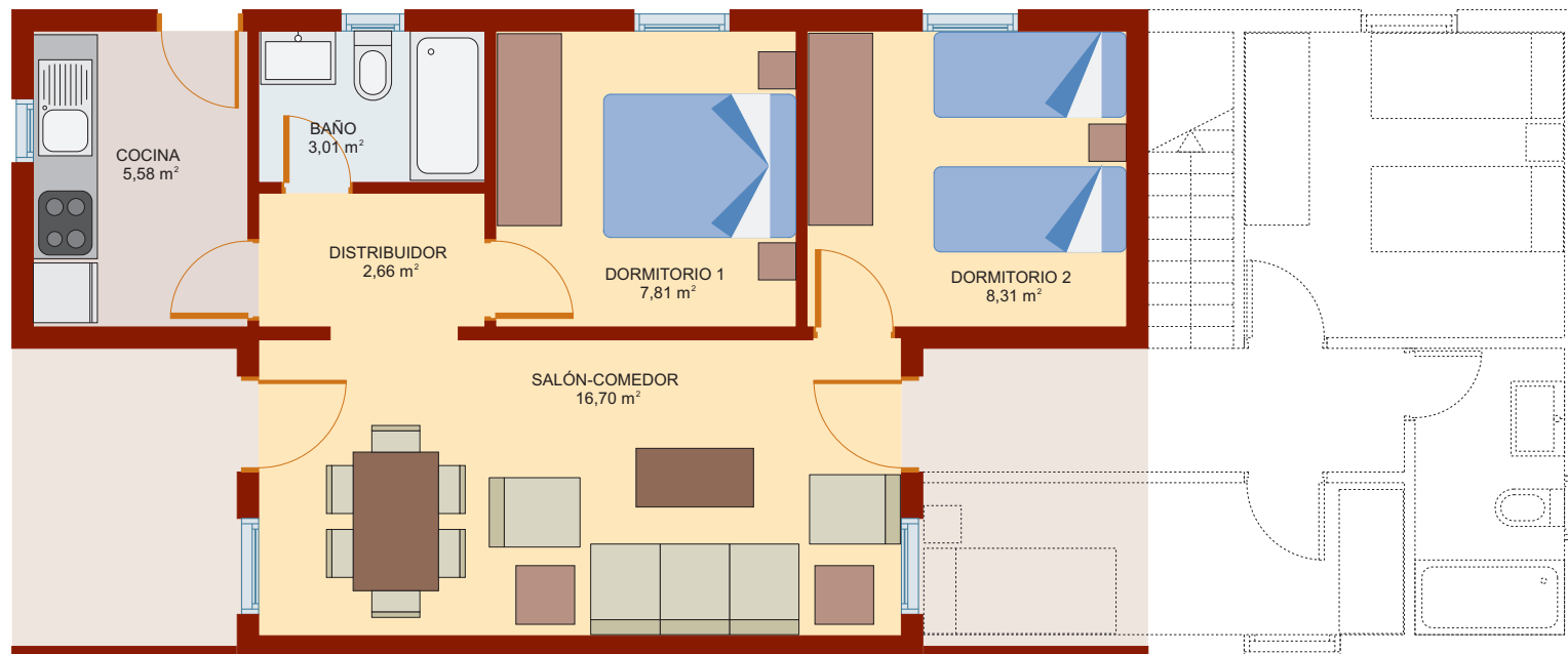
PLANTA TIPO
