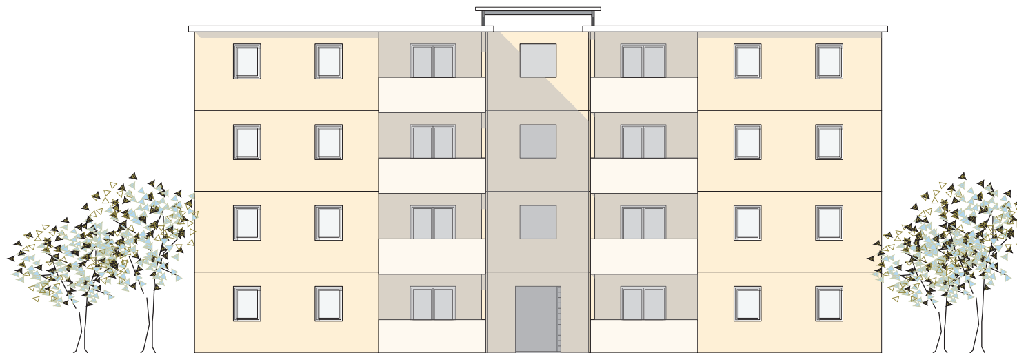
Alzado Frontal
