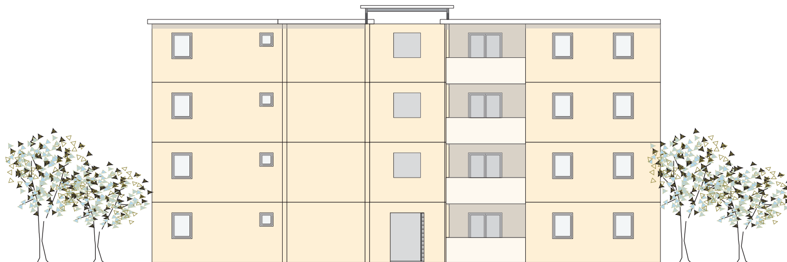
Alzado Posterior
