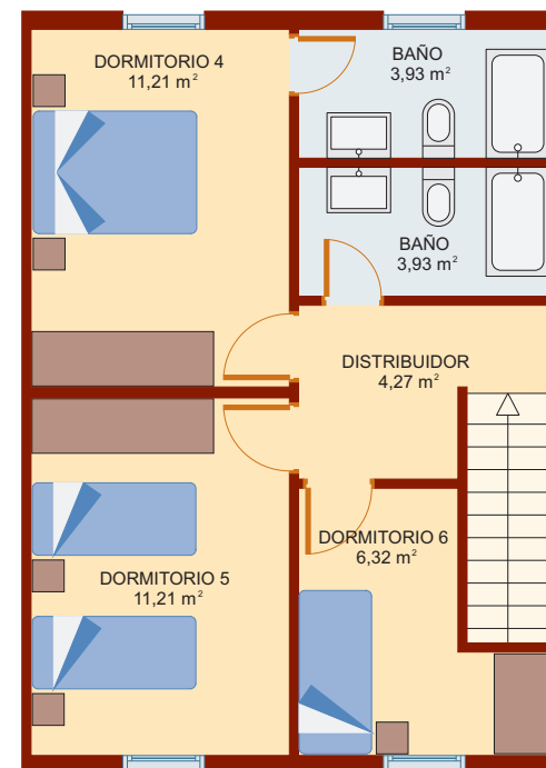
PLANTA PRIMERA
