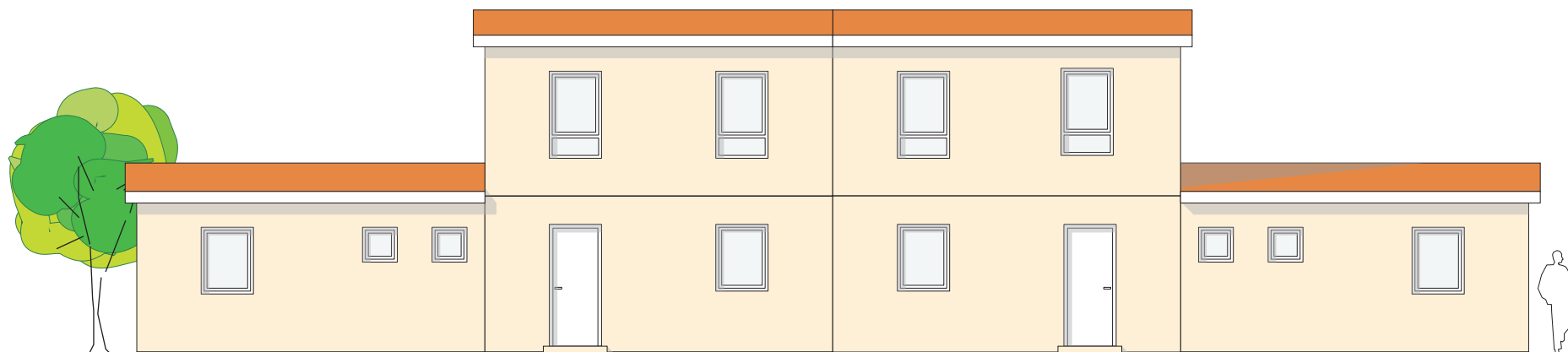
Alzado Posterior
