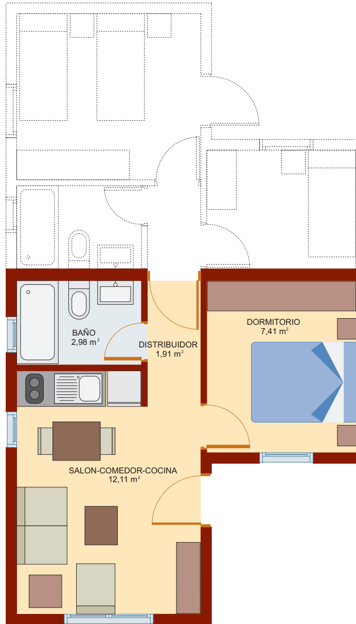
PLANTA TIPO
