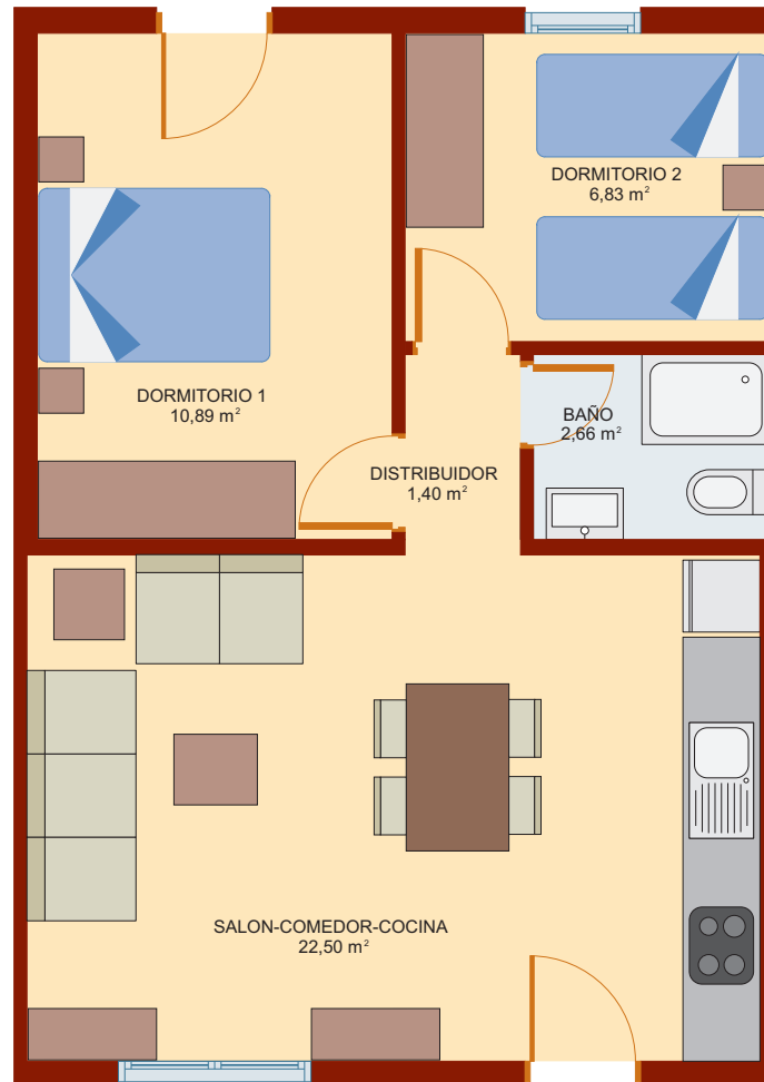
PLANTA TIPO
