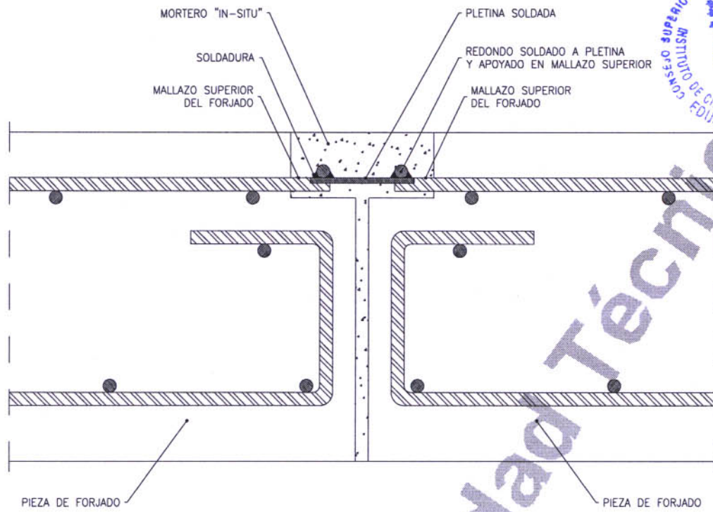
FIG.5 JUNTA HORIZONTAL DE UNION DE FORJADOS
