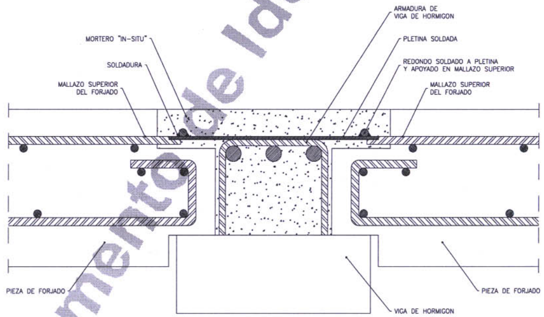
FIG.6 APOYO DE FORJADOS EN VIGA DE HORMIGON
