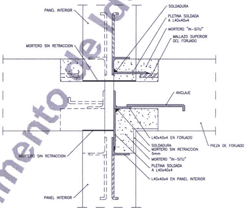
FIG.2 UNION DE PANELES INTERIORES CON FORJADOS
