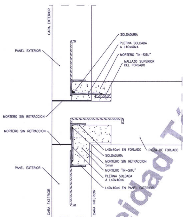
FIG.1 UNIONES DE PANELES EXTERIORES CON FORJADO
